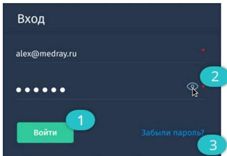
Окно «Авторизация»
